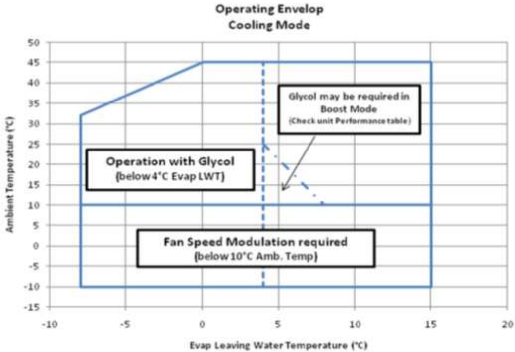
Abbildung 1 - Betriebsgrenzwerte bei Kühlen - EWYD-BZSS / EWYD-BZSL
