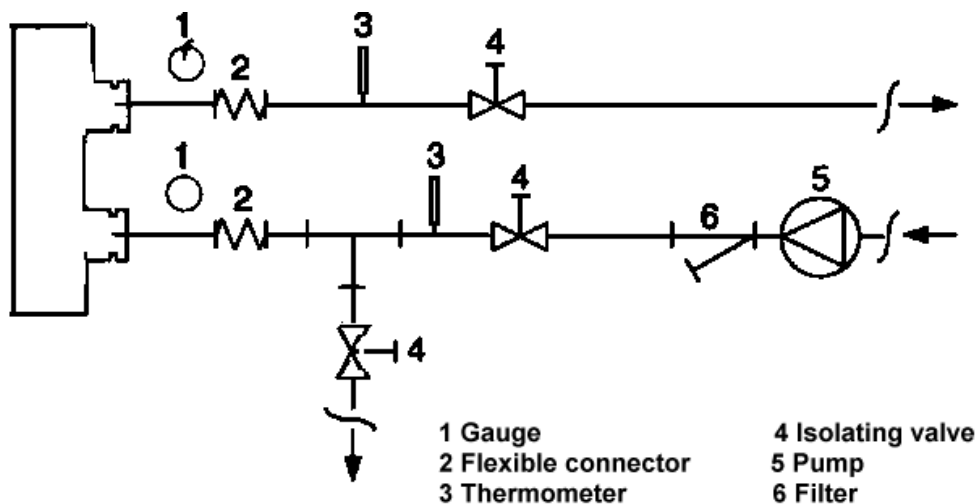
Abbildung 7 - Wasserrohranschlüsse für Wärmerückgewinnungs-Wärmetauscher
