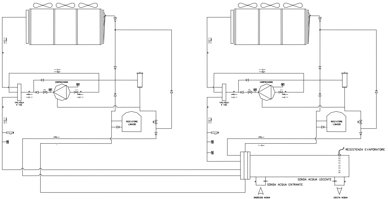
Abbildung 20 - Kältemittelkreislauf
