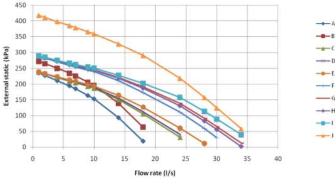
Abbildung 11 - Hochhub-Wasserpumpen-Kit (optional auf Anfrage) – Hub-Diagramme
