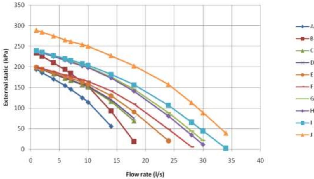
Abbildung 10 - Niederhub-Wasserpumpen-Kit (optional auf Anfrage) – Hub-Diagramme
