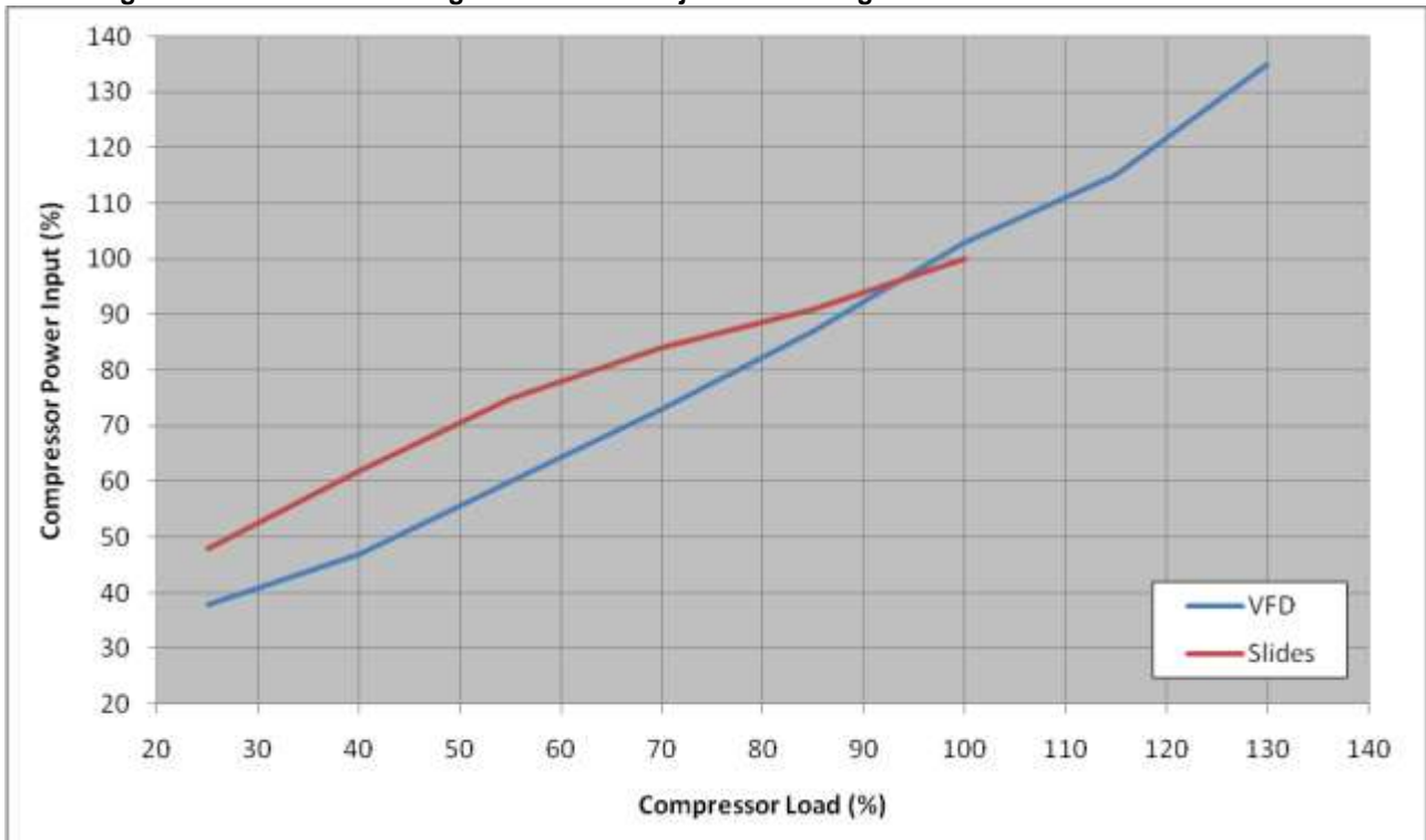
Abbildung 15 - Absorbierte Leistung des Verdichters je nach Ladung
