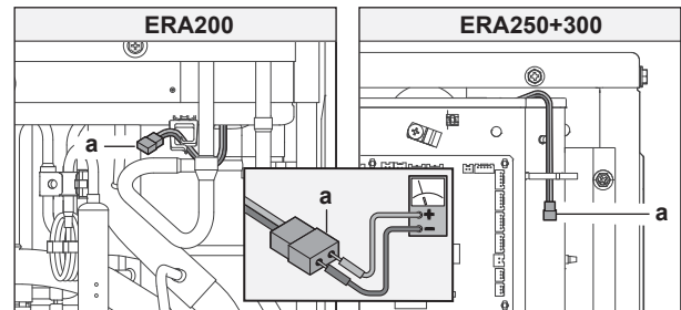
a Konnektor für Spannungsüberprüfung des Kondensators
