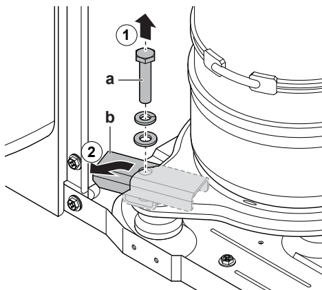
a Bolzen b Transportstütze
