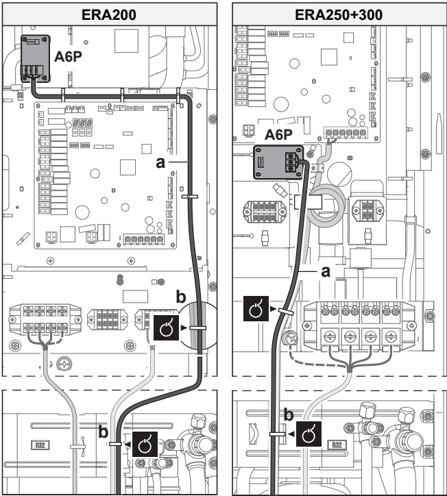
A6P Platine (Wahlschalter Kühlen/Heizen) a Kabel zu Wahlschalter Kühlen/Heizen (KRC19-26A) b Kabelbinder
