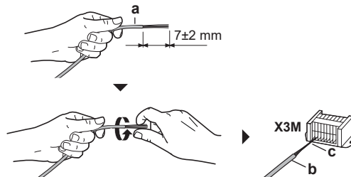
7–2 Das Kabel abschneiden und verdrehen und dann an der Klemmleiste anschließen.
