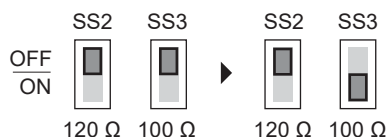
8-2 Beispiel: Schiebeschalter-Einstellungen wenn Widerstand 100 Ω ist
