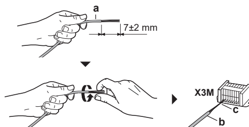
▲ 7-1 Das Kabel abschneiden und verdrehen und dann an der Klemmleiste anschließen.
