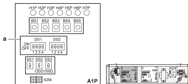
a DIP-Schalter (DS1, DS2)
