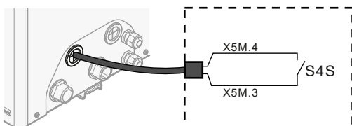
S4S Smart Grid-Impulszähler (optional)
