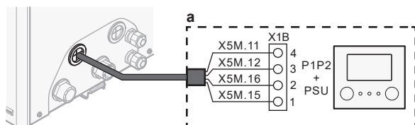
a Raumbedienmodul: für den Betrieb erforderlich. Wird als Zubehör mit dem Gerät ausgeliefert.
