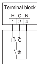
Thermostat Heizen/Kühlen
