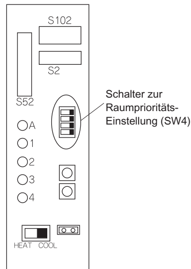
Wartungs-PCB
