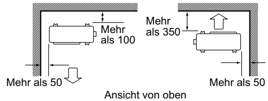
Bei Wänden an zwei Seiten
