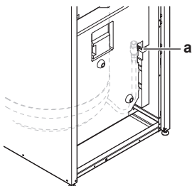
a Ablaufschlauch
