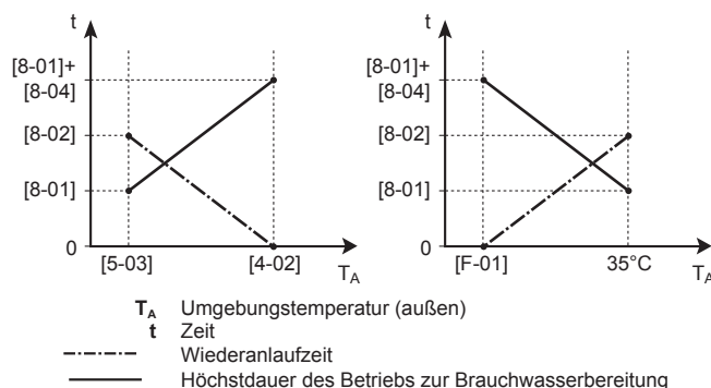
[8-04]: Zusätzliche Laufzeit bei [4-02]/[F-01]
