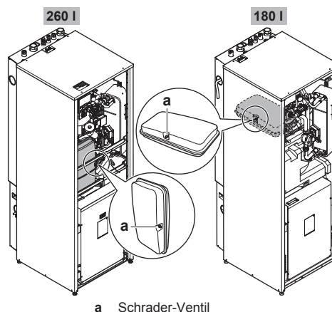
a Schrader-Ventil
