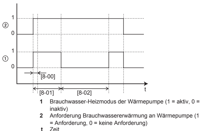
[8-03]: Verzögerungs-Timer der Zusatzheizung
