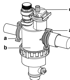
a Clip b Magnetischer Filter/Schmutzfilter c Entlüftungsventil
