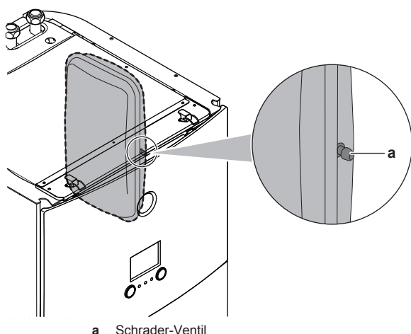
a Schrader-Ventil
