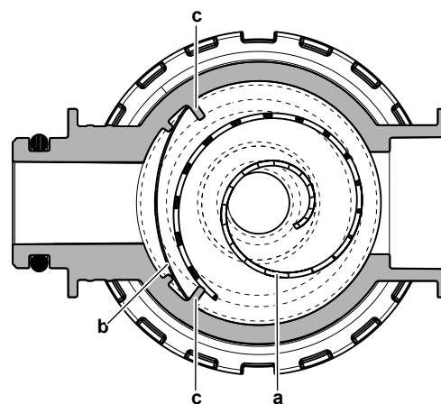
a Aufgerollter Filter b Sieb c Vorsprung
