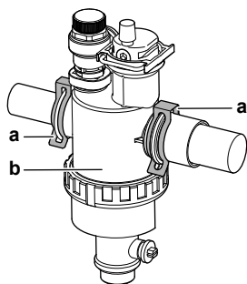
a Clip b Magnetischer Filter/Schmutzfilter
