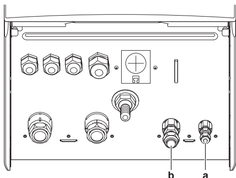
a Anschluss für flüssiges Kältemittel b Anschluss für gasförmiges Kältemittel
