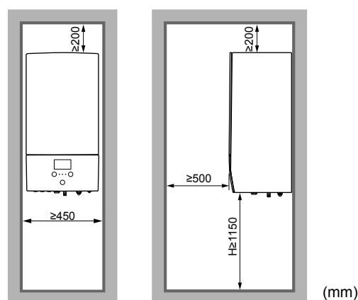
H Höhe gemessen von der Unterseite des Gehäuses bis zum Boden
