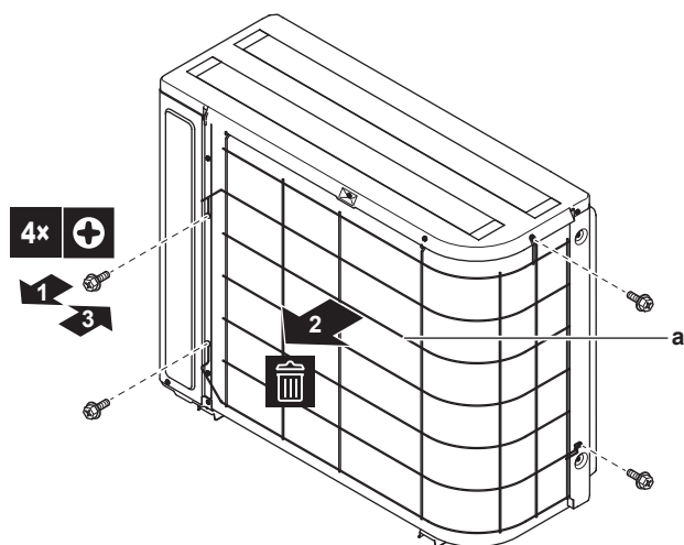
a Ansaugluftgitter
