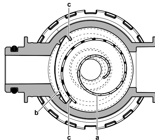
a Aufgerollter Filter b Sieb c Vorsprung
