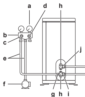
a Druckmesser b Mehrzweckmanometer c Niederdruckventil (Lo) d Hochdruckventil (Hi) e Füllschläuche f Vakuumpumpe g Wartungsanschluss h Ventildeckel i Gasleitungs-Absperrventil
