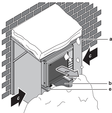
a Schneeabdeckung oder Unterstand b Untergestell c Vorherrschende Windrichtung d Luftauslass e Options-Kit EKFT008D
