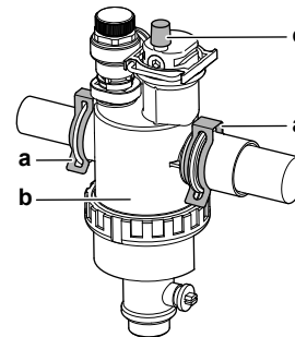
a Clip b Magnetischer Filter/Schmutzfilter c Entlüftungsventil
