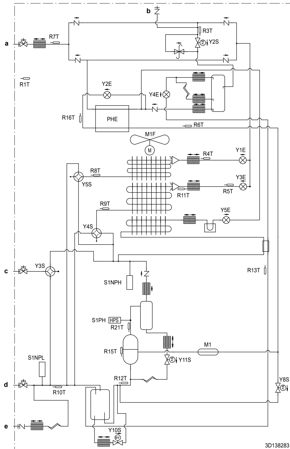
Rohrleitungsplan: 5~12 HP
